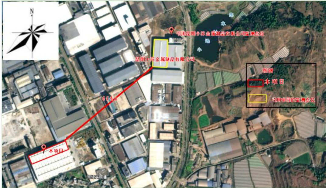
图 3-3 项目的监测点位图
