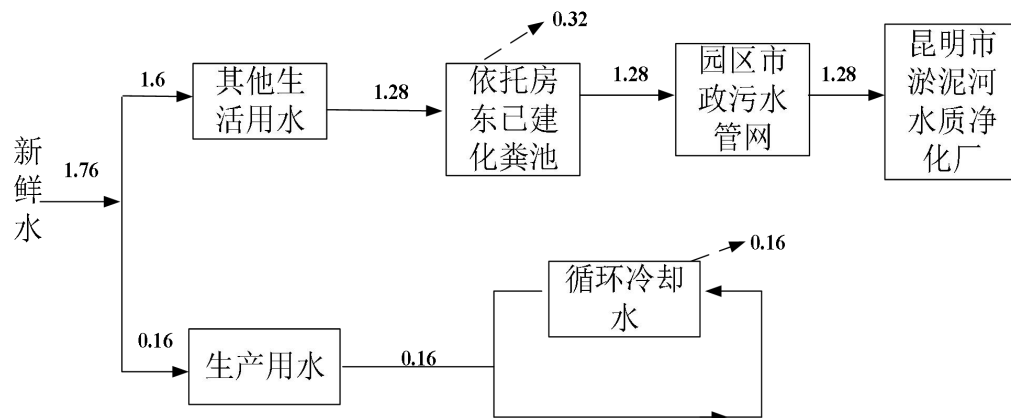
图 2-1 项目水量平衡图单位： \text{m}^3/\text{d}
