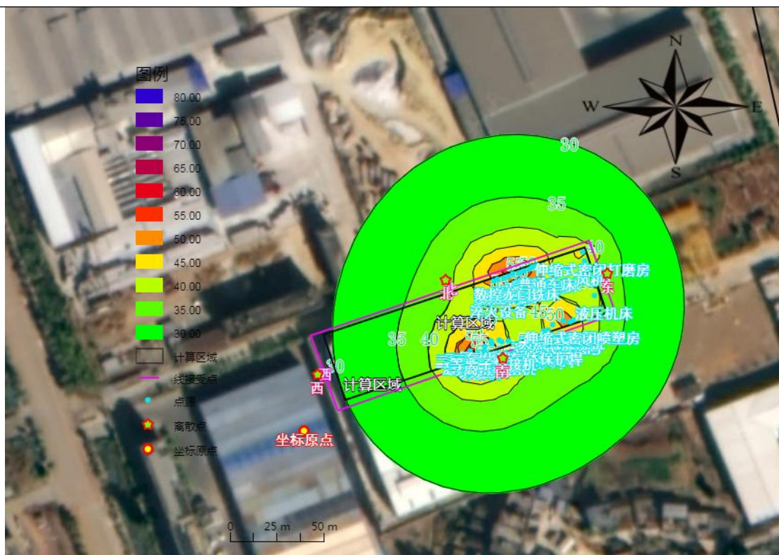
图 4-1 项目昼间等声值线图
