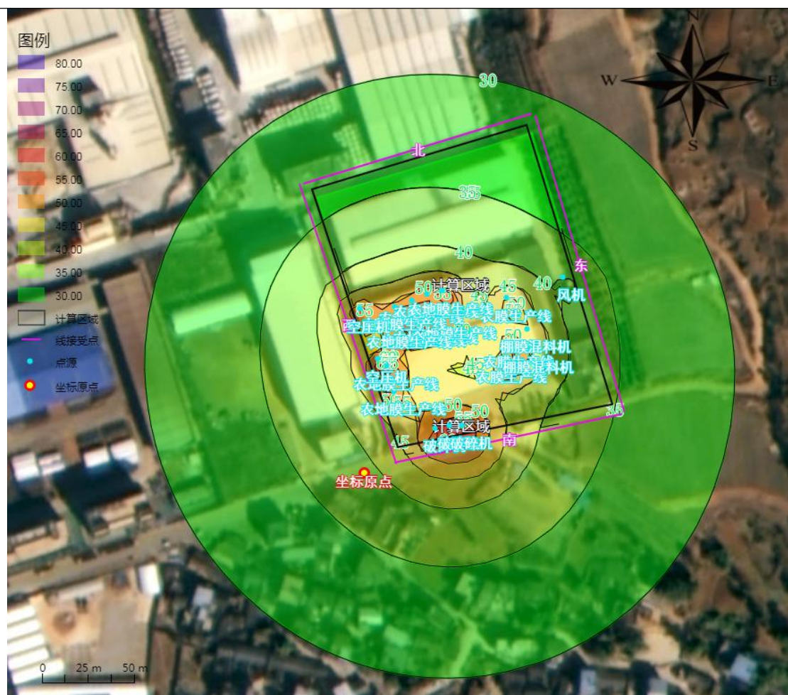
图 4-1 项目昼间等声值线图
