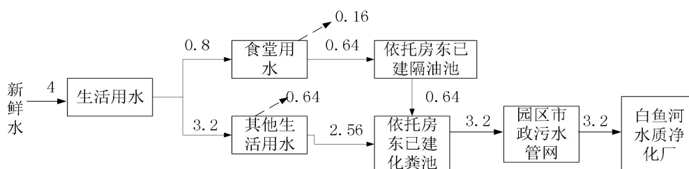
图 2-1 项目水量平衡图单位： \text{m}^3/\text{d}
