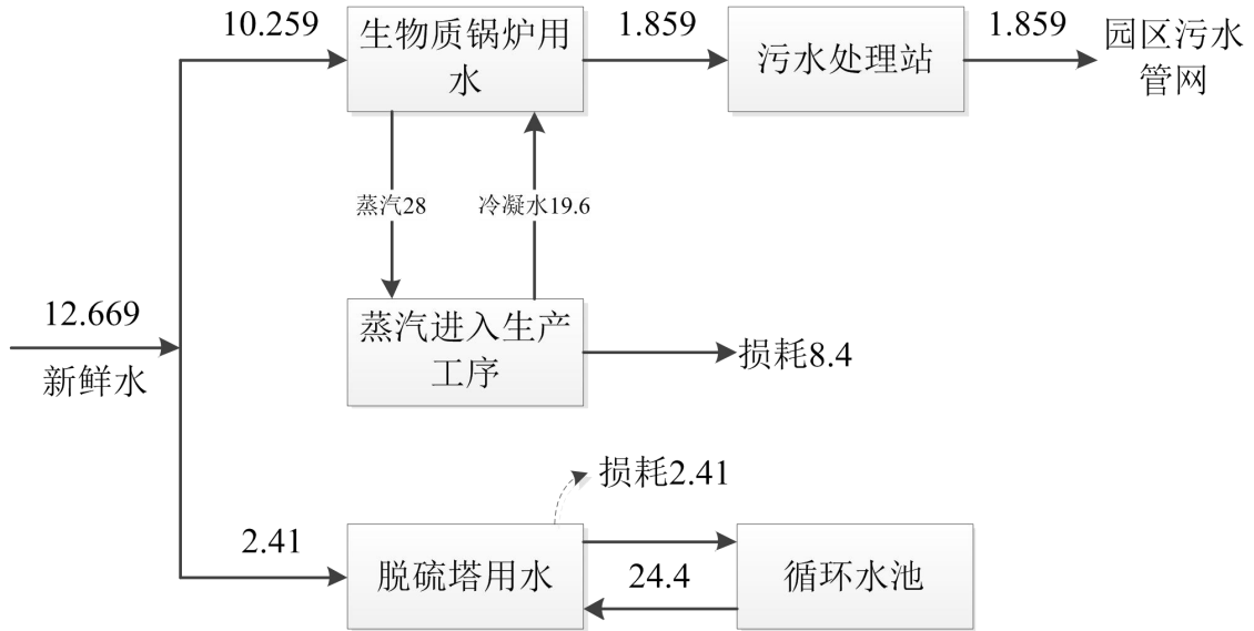
图 2-2 改建项目水量平衡图 单位: m 3 /d
