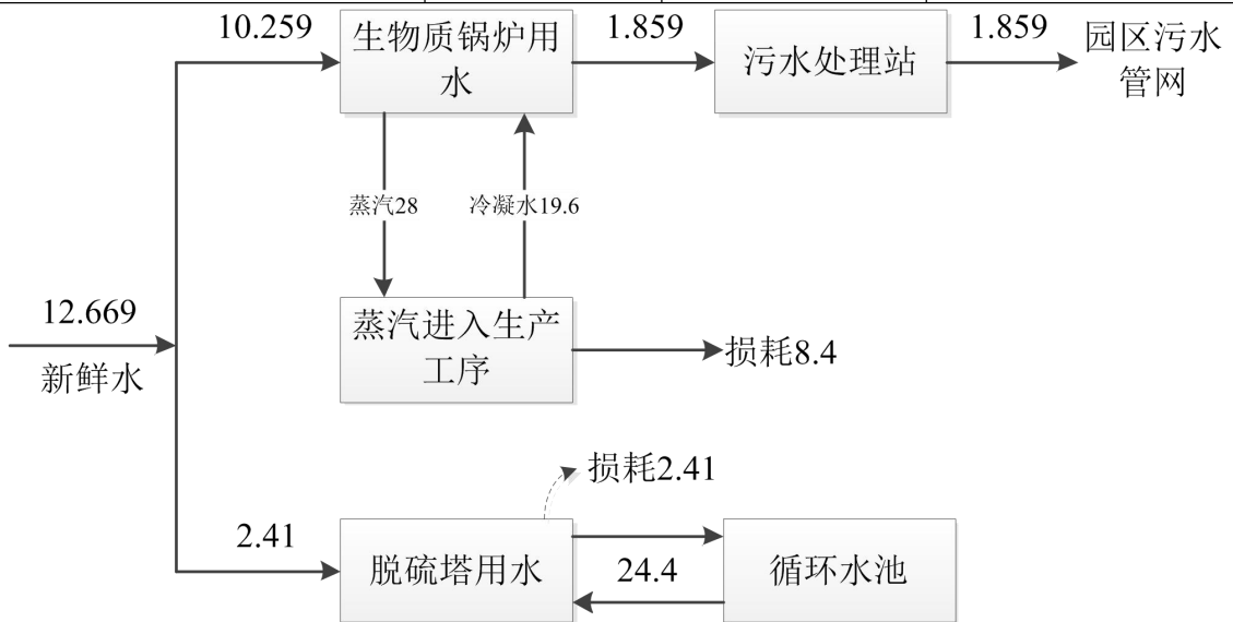
图 4-1 项目运营期水量平衡图 单位：m 3 /d
