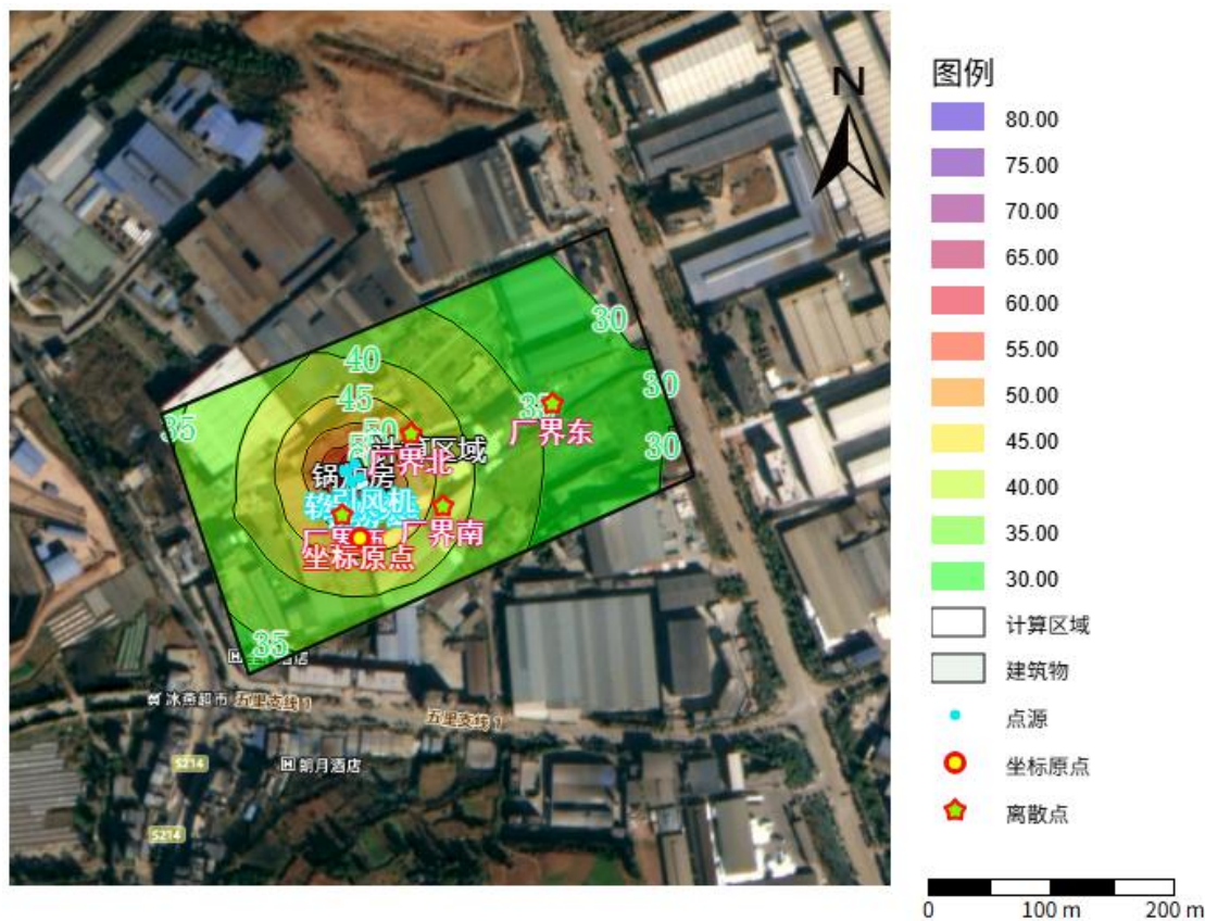
图 4-2 本项目厂界噪声（昼间）等值线图
