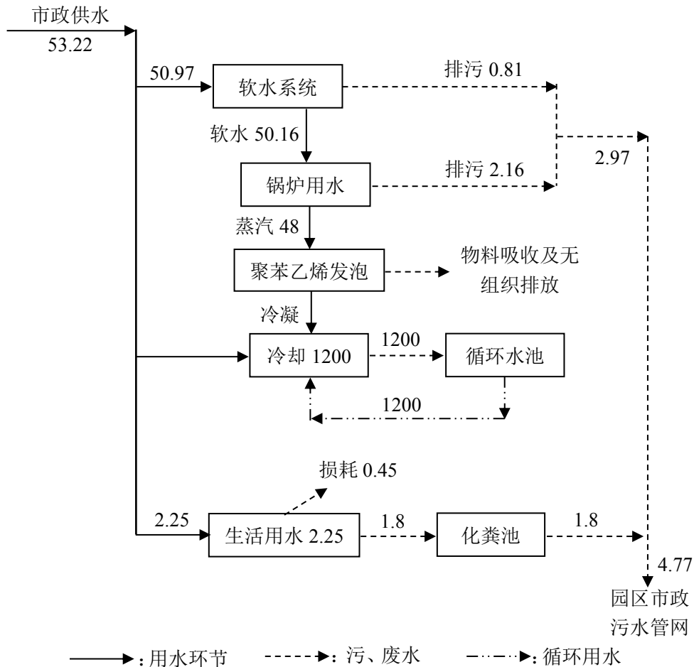
图 2-2 项目实施后全厂水量平衡图 单位：m 3 /d
