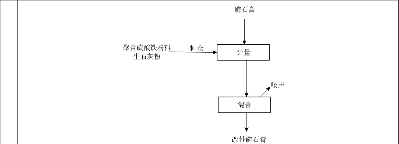
图 2-8 改性磷石膏工艺流程及产污节点图
