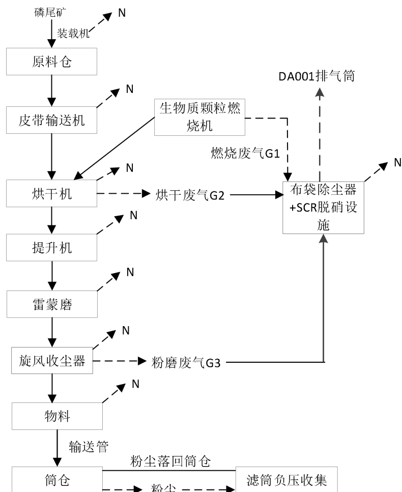
图2.12-2 磷尾矿烘干生产工艺流程及产污节点
