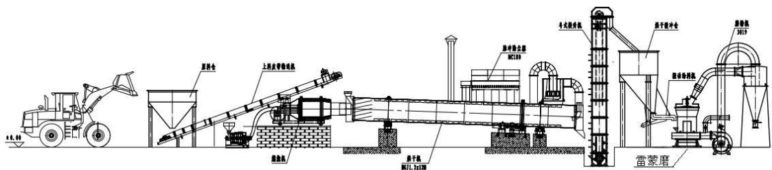
图 2.6-1 磷尾矿烘干系统示意图
