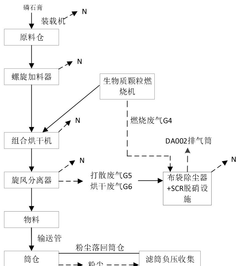
图2.12-3 磷石膏烘干生产工艺及产污节点图
