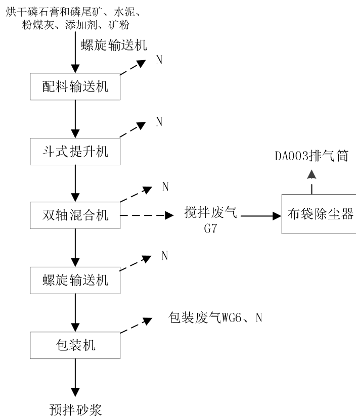
图2.12-5 预拌砂浆生产工艺流程及产污节点图
