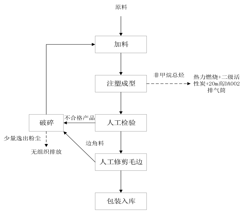
图 2-3 项目塑料包装箱工艺流程及产污节点图
