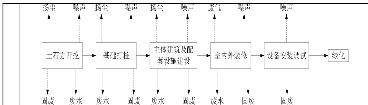
图 2-1 项目施工期工艺流程及产污节点图
