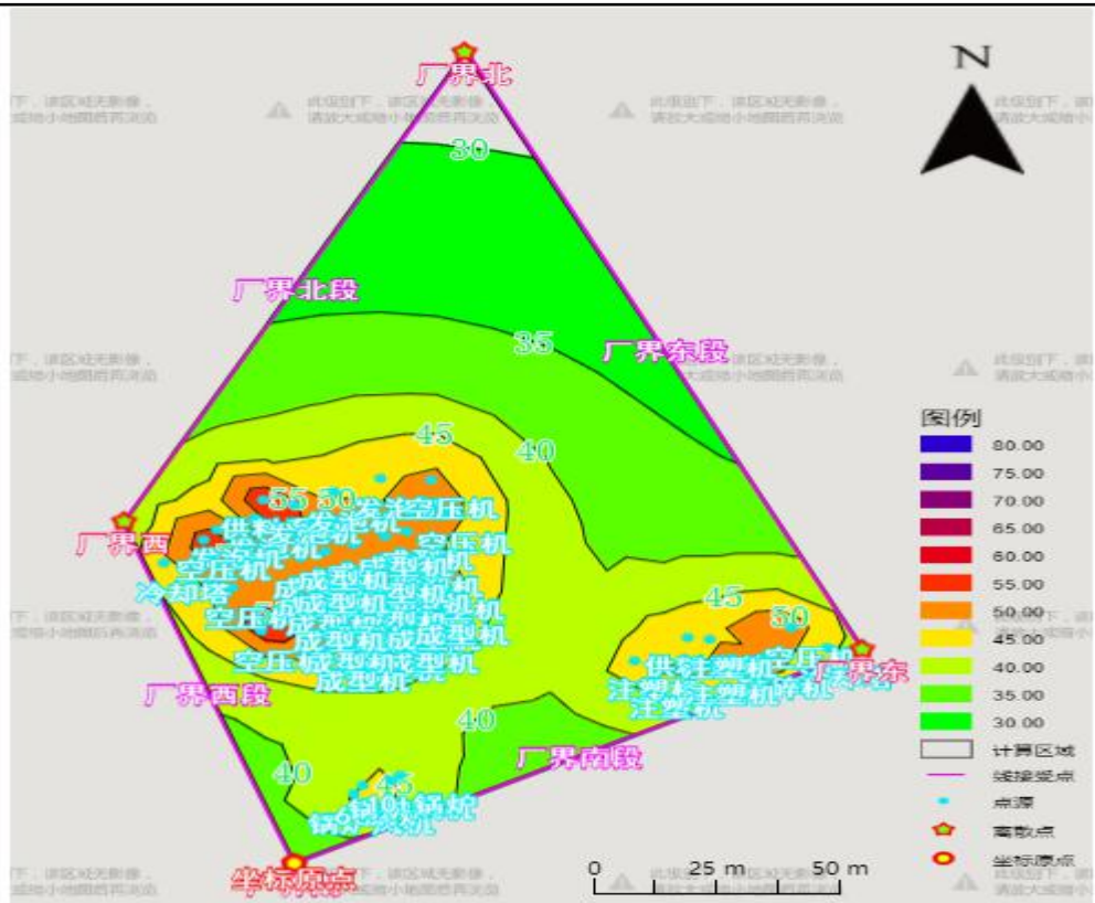
图 4-2 项目等声值线图
