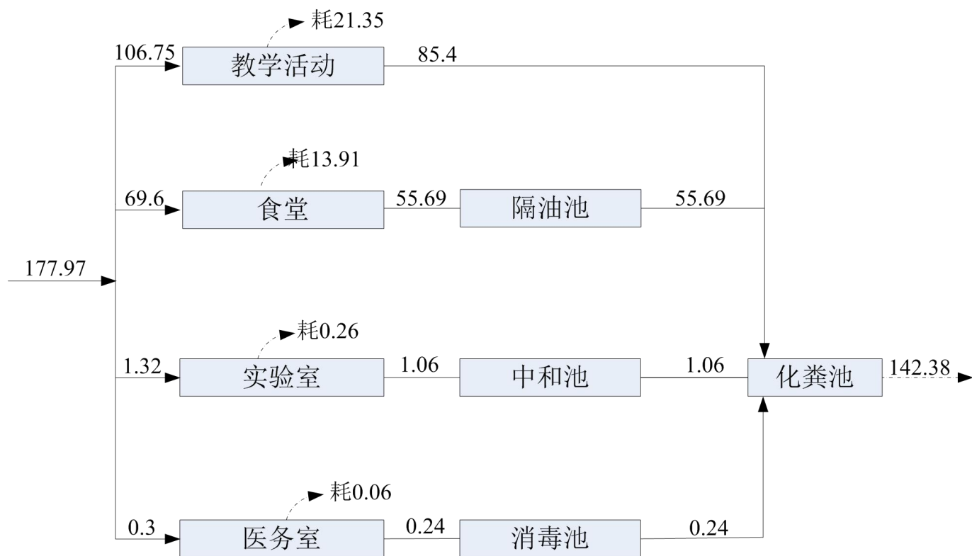
图 4-2 雨天水量平衡图 单位: m³/d
