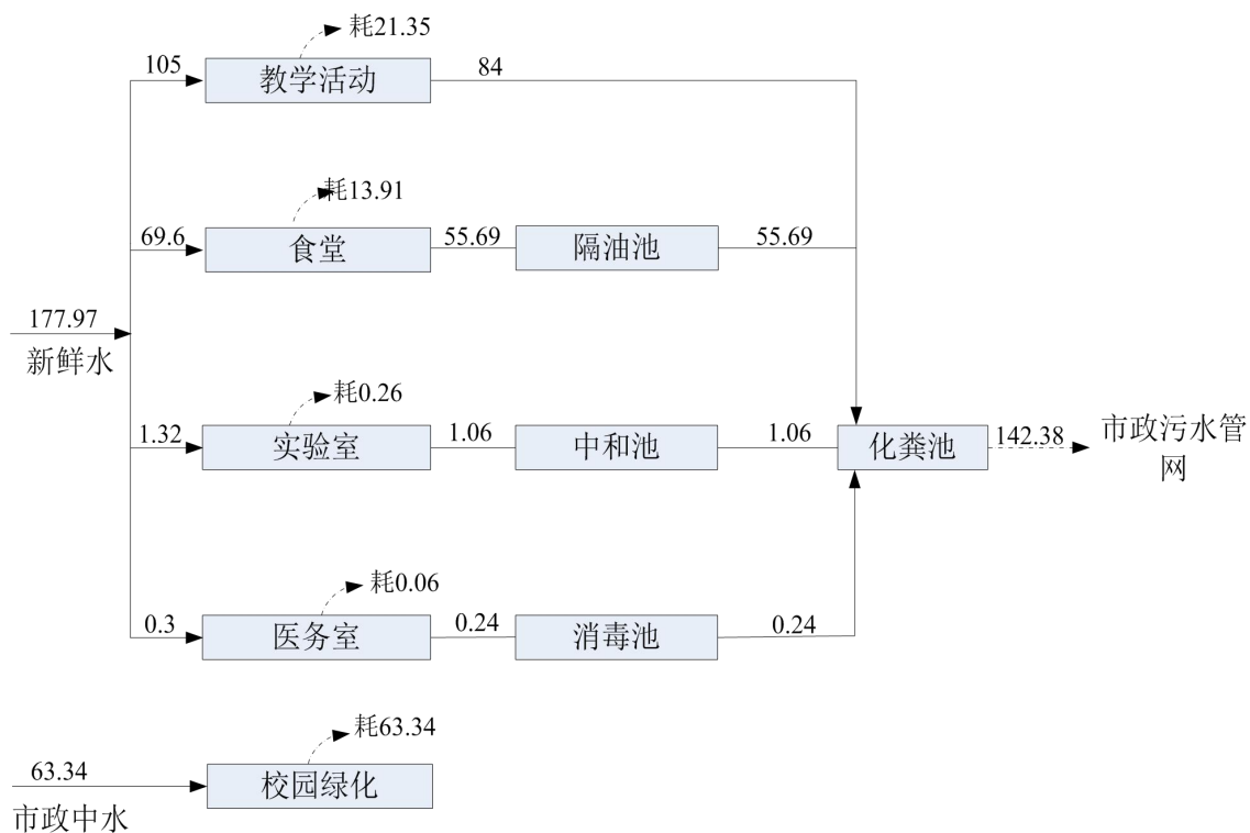
图 4-1 晴天水量平衡图 单位: m³/d
