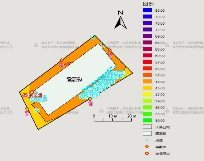
图 4-1 项目昼间等声值线图
