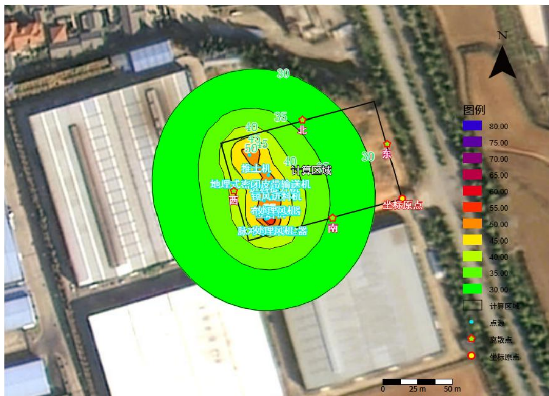
图 4-1 项目昼间等声值线图
