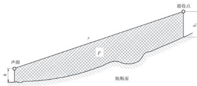
图 17 估计平均高度 h_m 的方法
