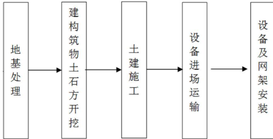
图 6 变电站主变扩建工程施工工艺流程
