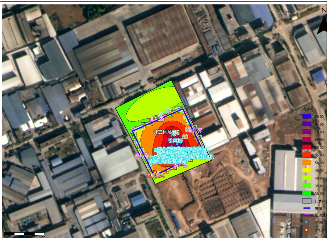
图 4-2 项目噪声预测等值线图 表 4-17 厂界噪声预测结果单位: dB(A)
