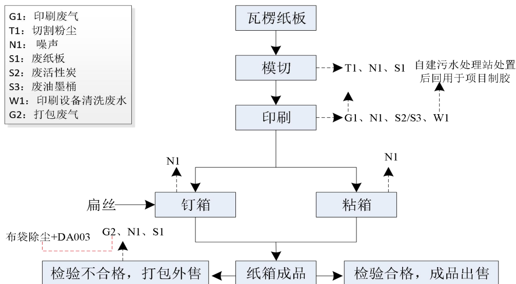
图2-4 瓦楞纸箱生产工艺流程及产污节点图
