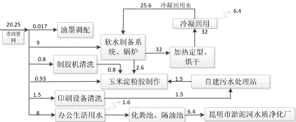
图 2-1 本项目水平衡图 (m 3 /d)
