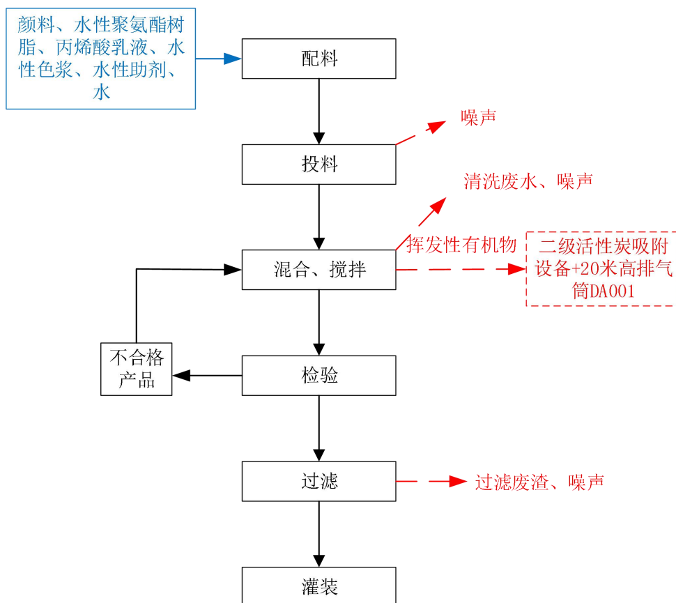
图2-3水性新材料生产线工艺及产污节点图
