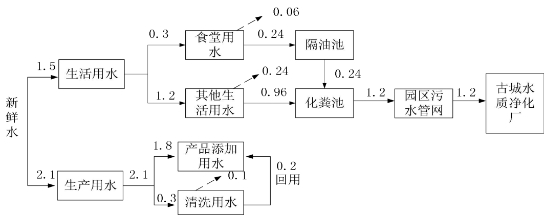
图2-1项目水量平衡图 单位：m³/d
