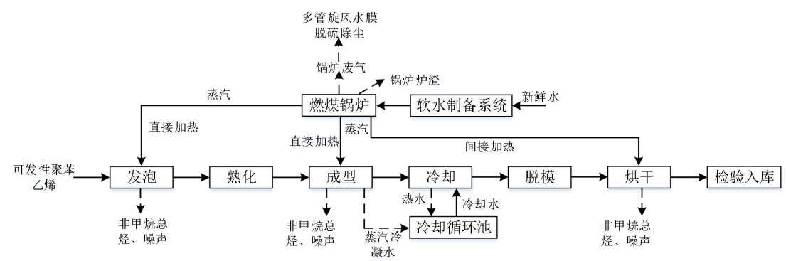
图 2-4 原有项目泡沫塑料制品生产工艺及产污环节图
