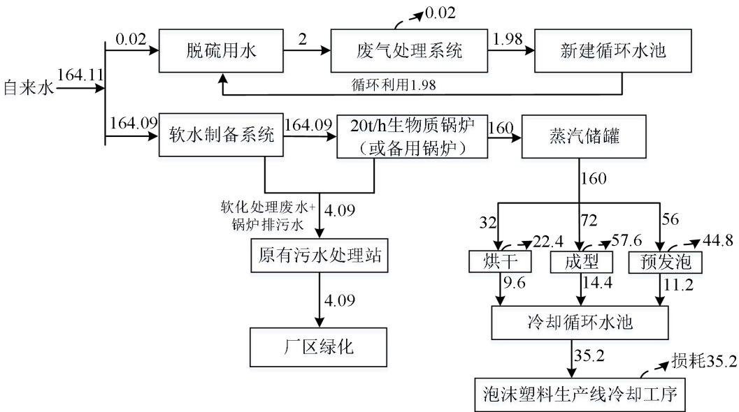
图 2-2 项目水平衡图（m³/d）
