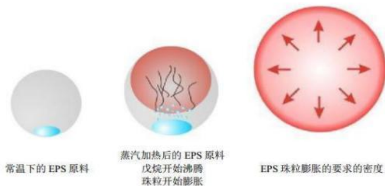
图 2-5 可发性聚苯乙烯珠粒发泡示意图
