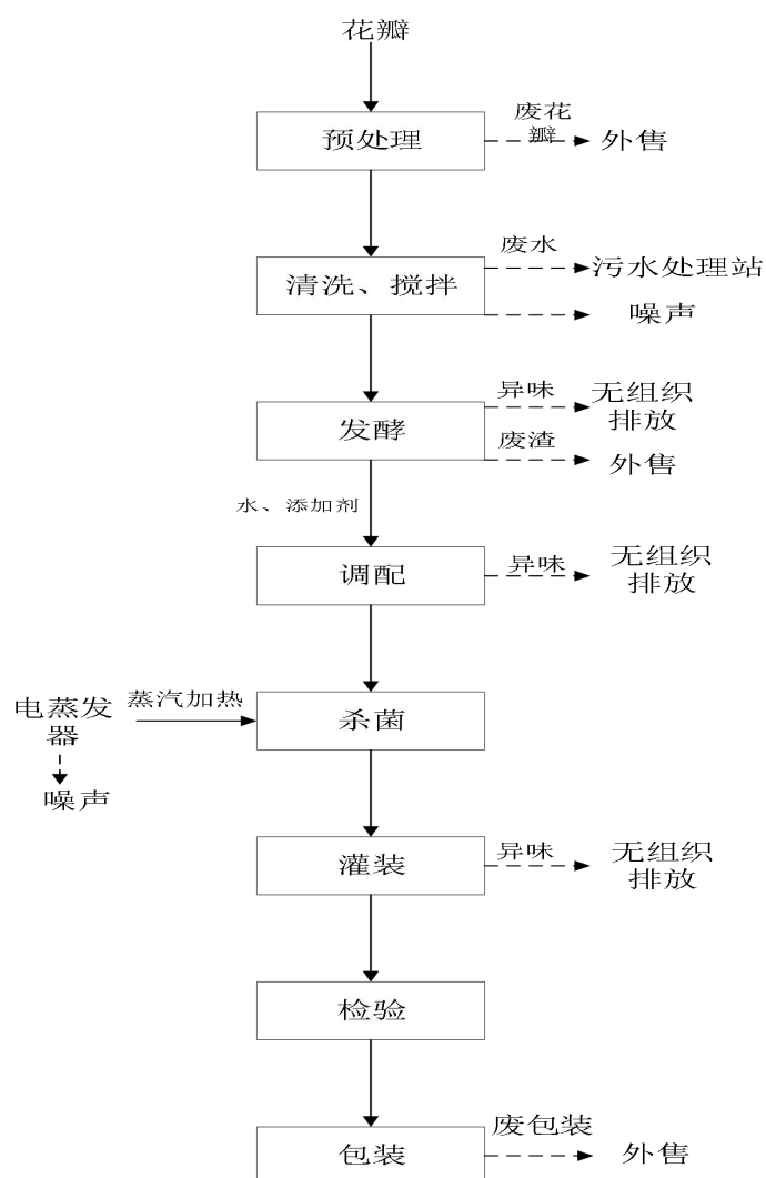
图 2-3 玫瑰花醋生产工艺流程及产污节点图
