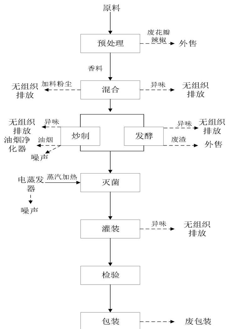
图 2-6 辣酱生产工艺流程及产污节点图
