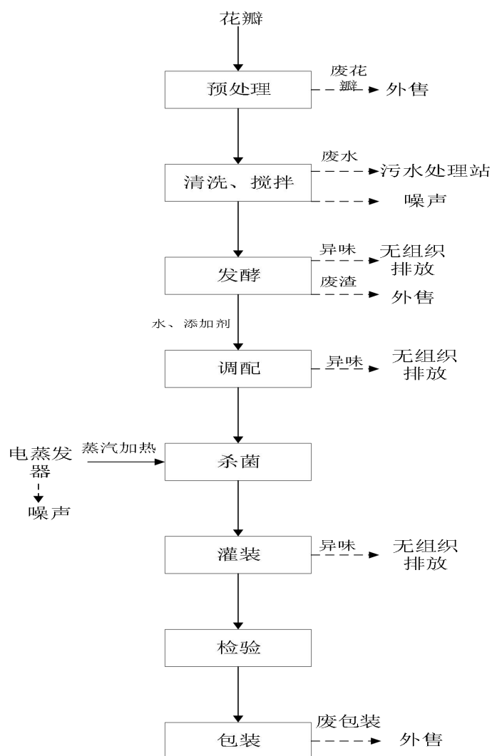
图 2-4 玫瑰花汁生产工艺流程及产污节点图
