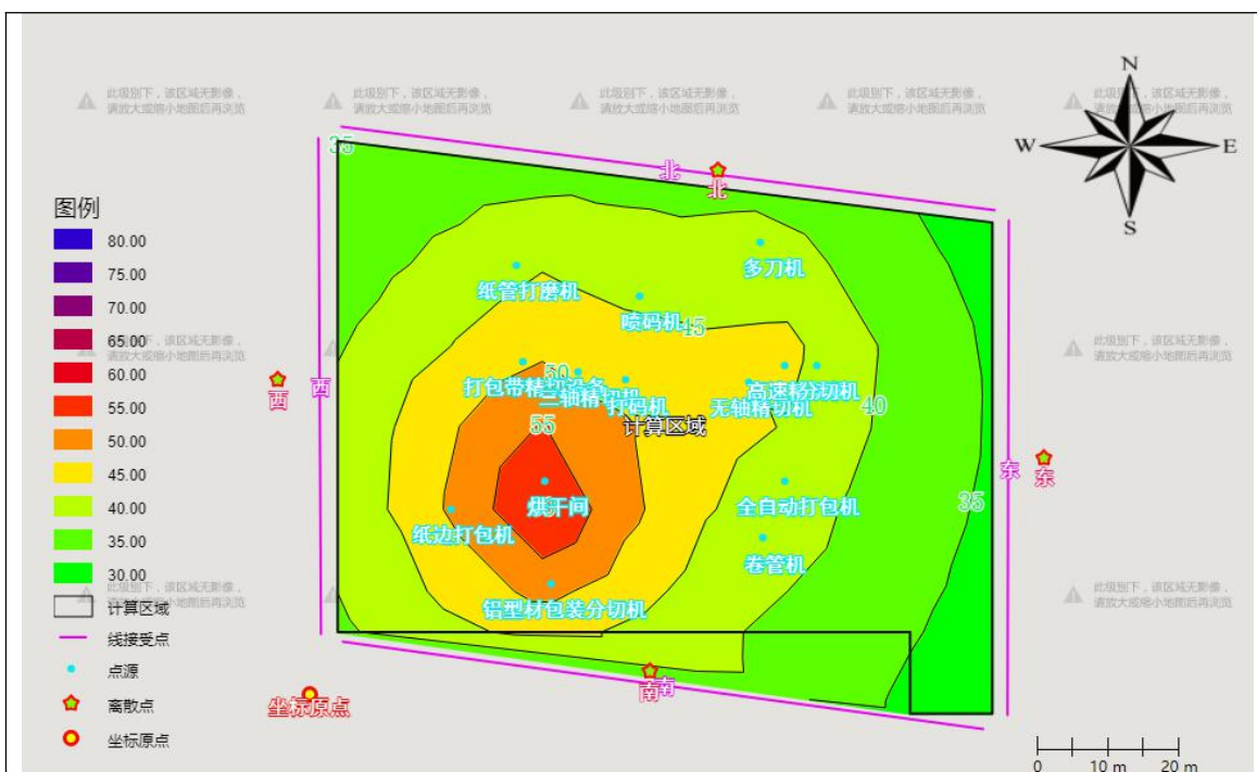
图 4-18 项目昼间等声值线图
