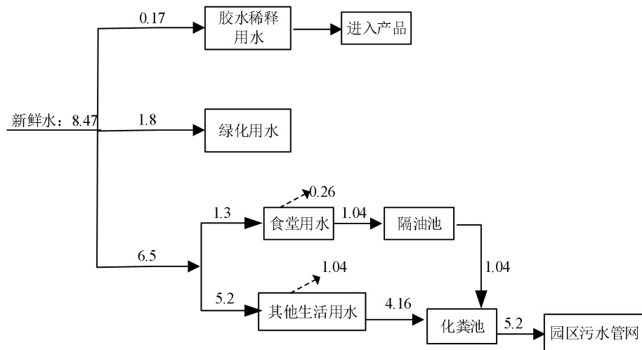
图 4-13 项目用水产出流程图（单位：m³/d）
