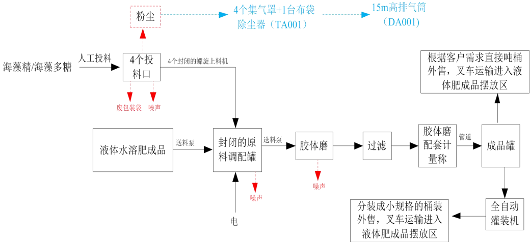
图 2-4 液体海藻水溶肥生产工艺流程及产污环节
