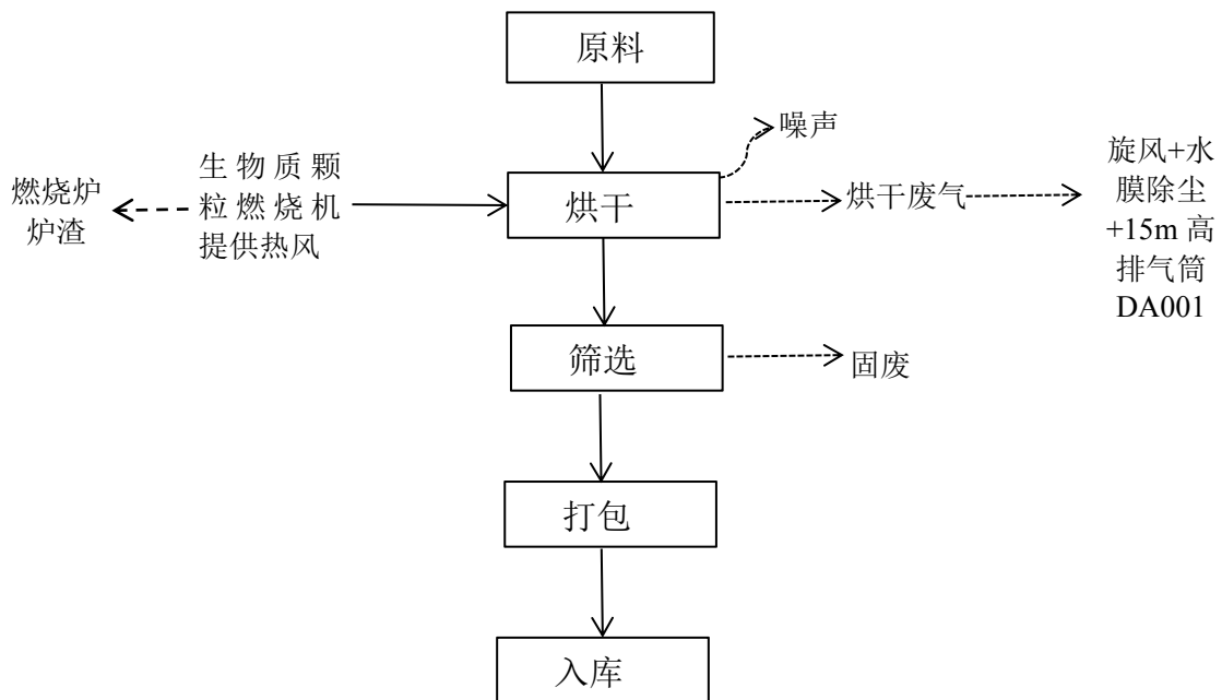
图 2-4 食用野生菌、花生烘干工艺流程及产污节点图
