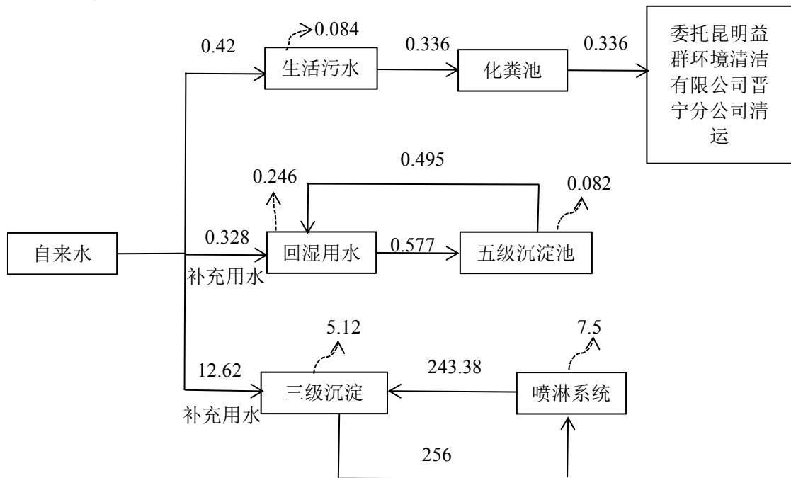
图 2-1 项目用水量平衡图 单位 m 3 /d
