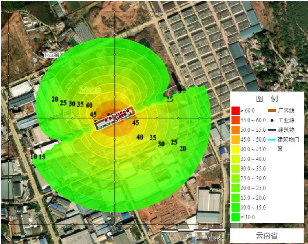
图 4-3 项目昼间等声值线图
