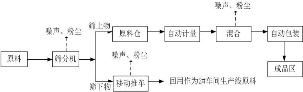
图 2-1 掺混肥料生产工艺流程图
