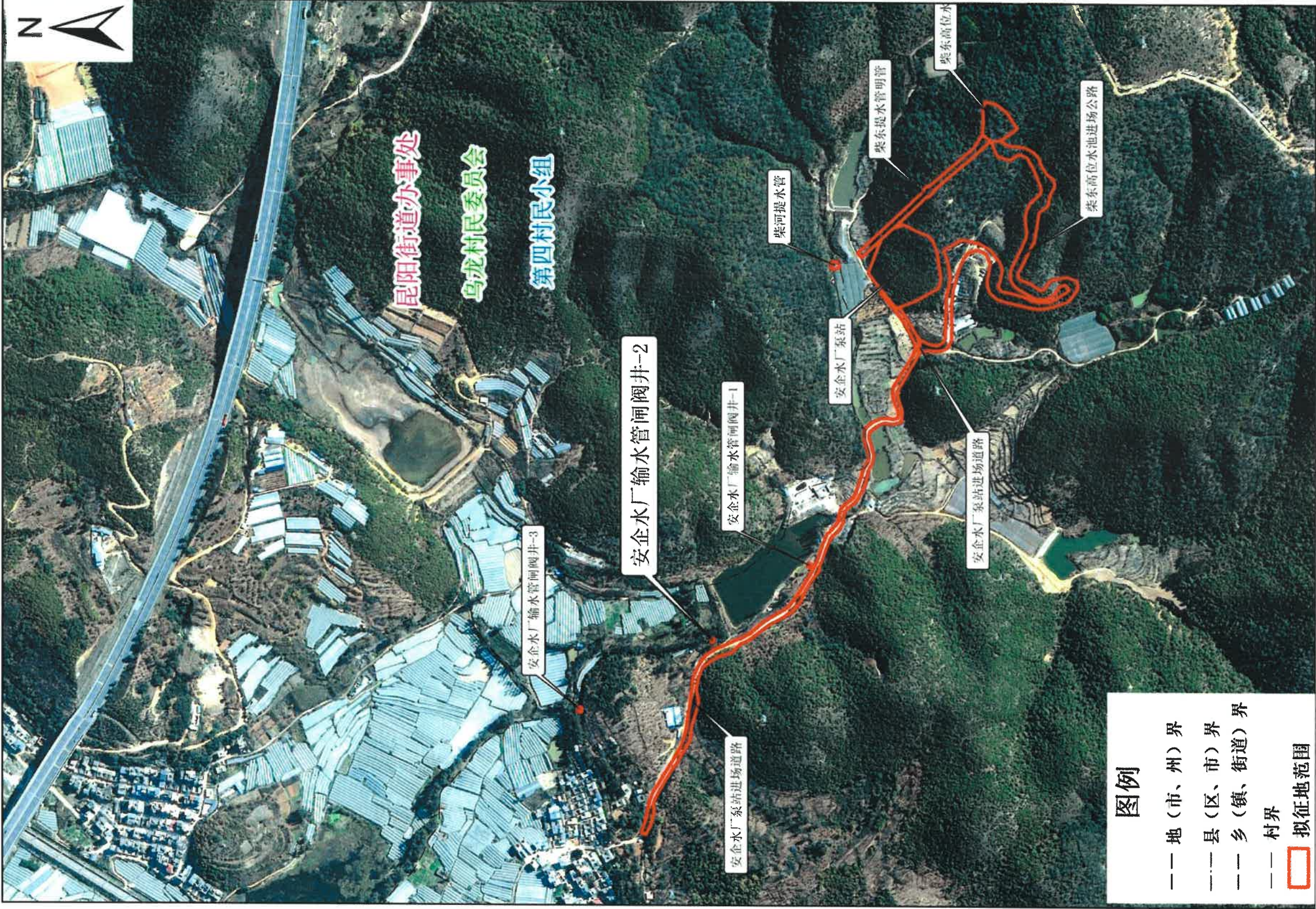
云南省滇中引水二期配套工程建设项目（昆明市晋宁区段）拟征收土地示意图(7)
