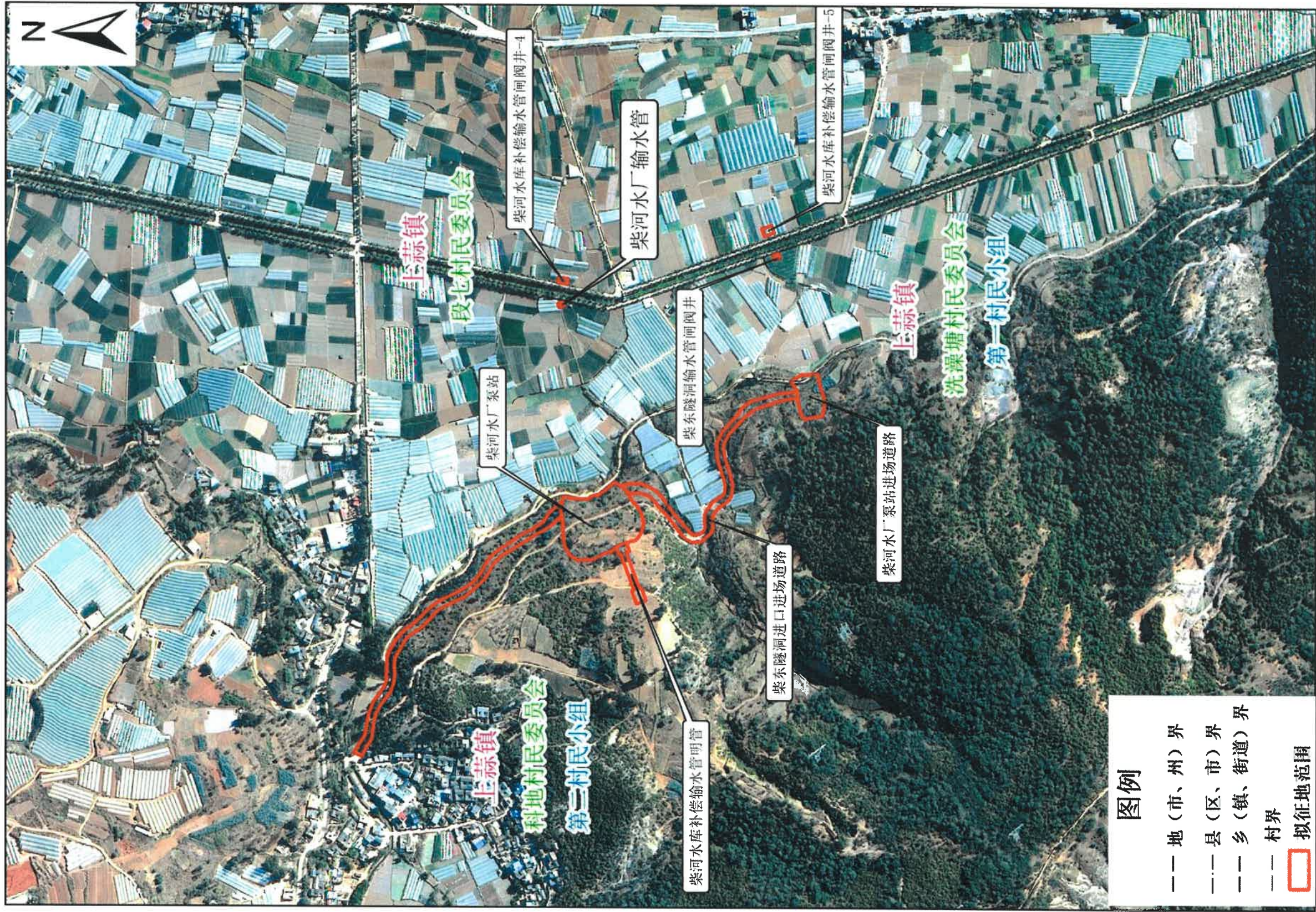
云南省滇中引水二期配套工程建设项目（昆明市晋宁区段）拟征收土地示意图（10）
