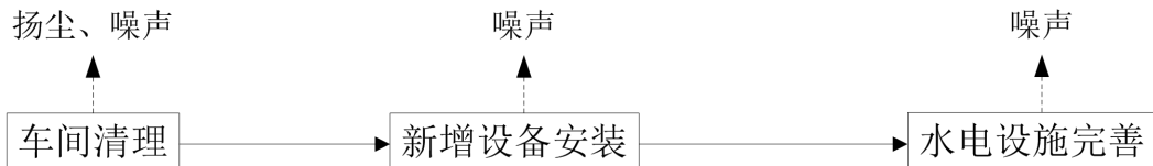
图 2-1 项目施工期工艺流程及产污节点图
