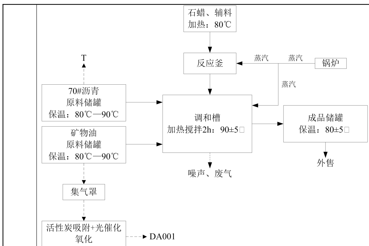
图 2-1 项目工艺流程及产污节点图
