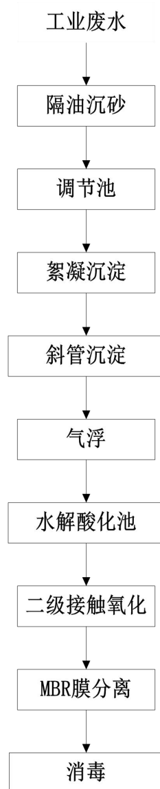
图 4-1 园区工业废水处理站工艺流程
