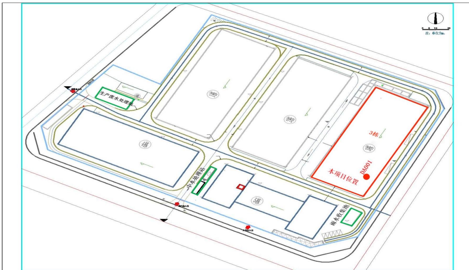
附图5 厂区总平面布置图
