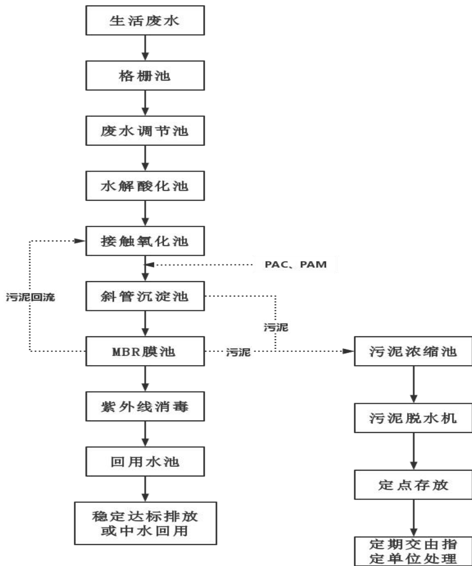
图 4-2 生活污水处理站工艺流程
