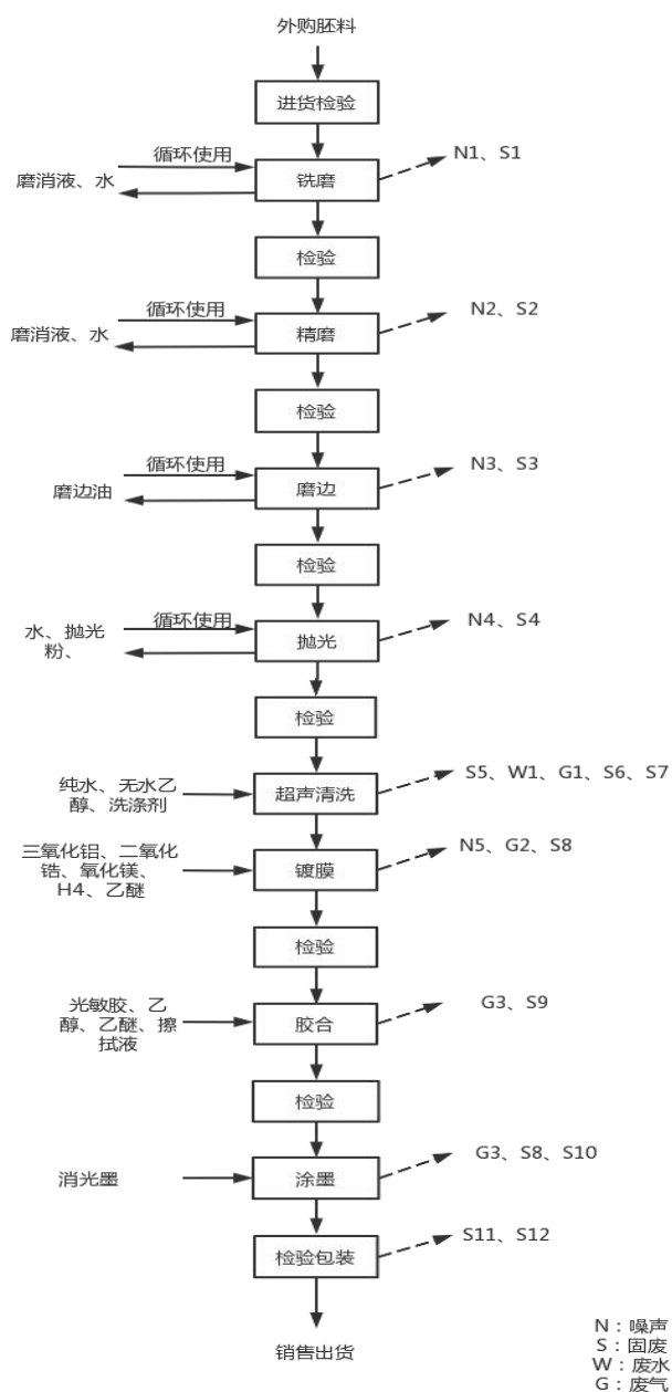
图 2-2 工艺流程图
