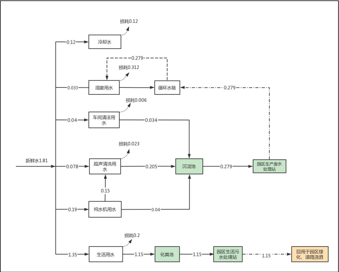
图 2-1 项目运营期水量平衡图 单位：m³/d
