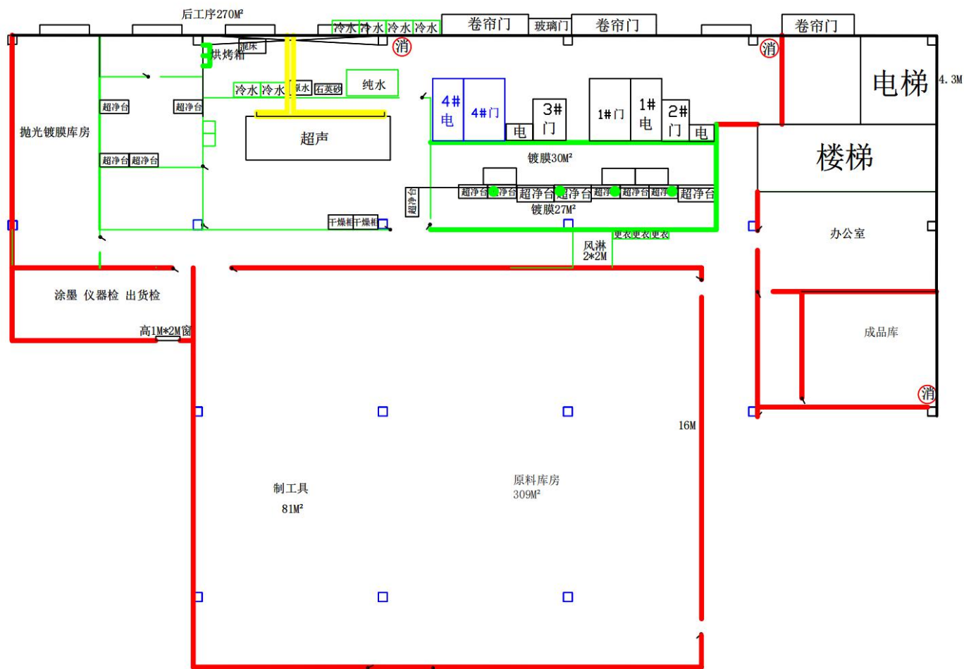
附图 6 工房总平面布置图
