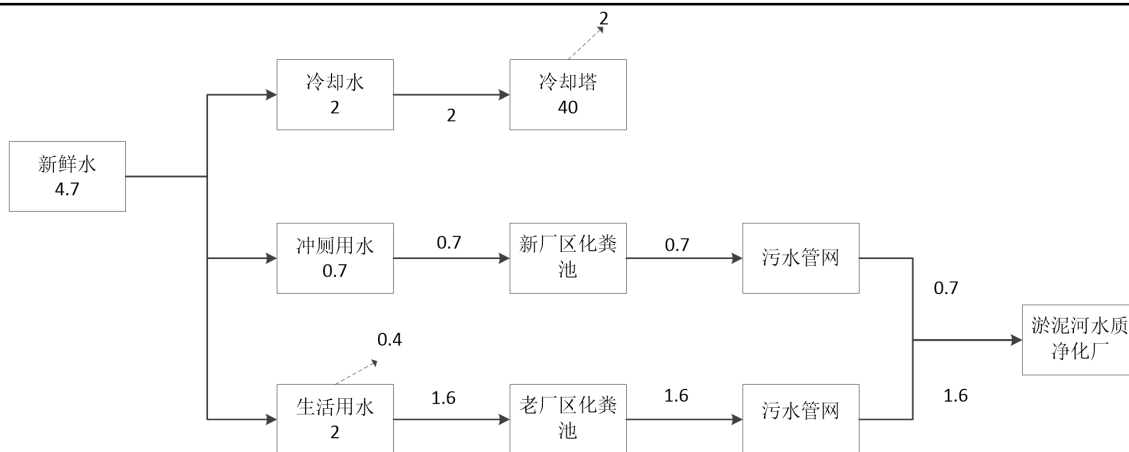
图 2-1 项目水量平衡图 (单位: m³/d)
