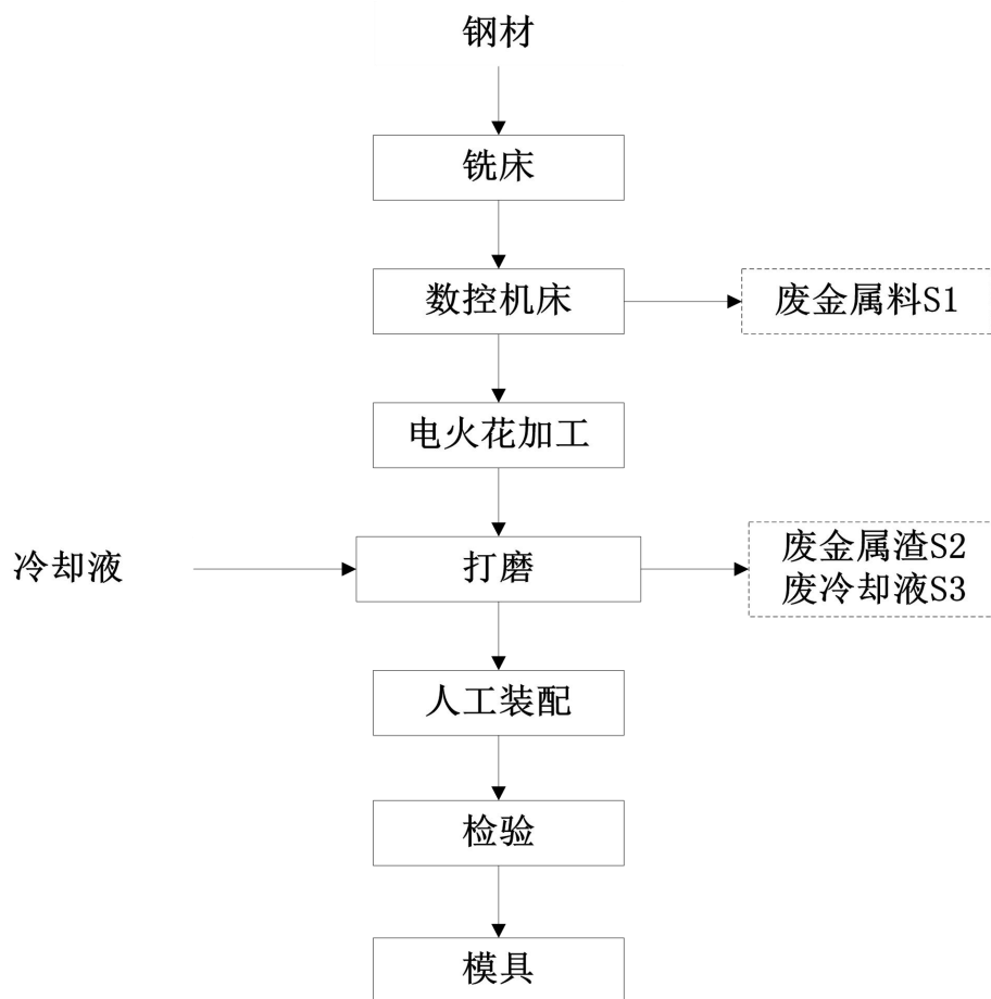
图 2-3 模具工艺流程图
