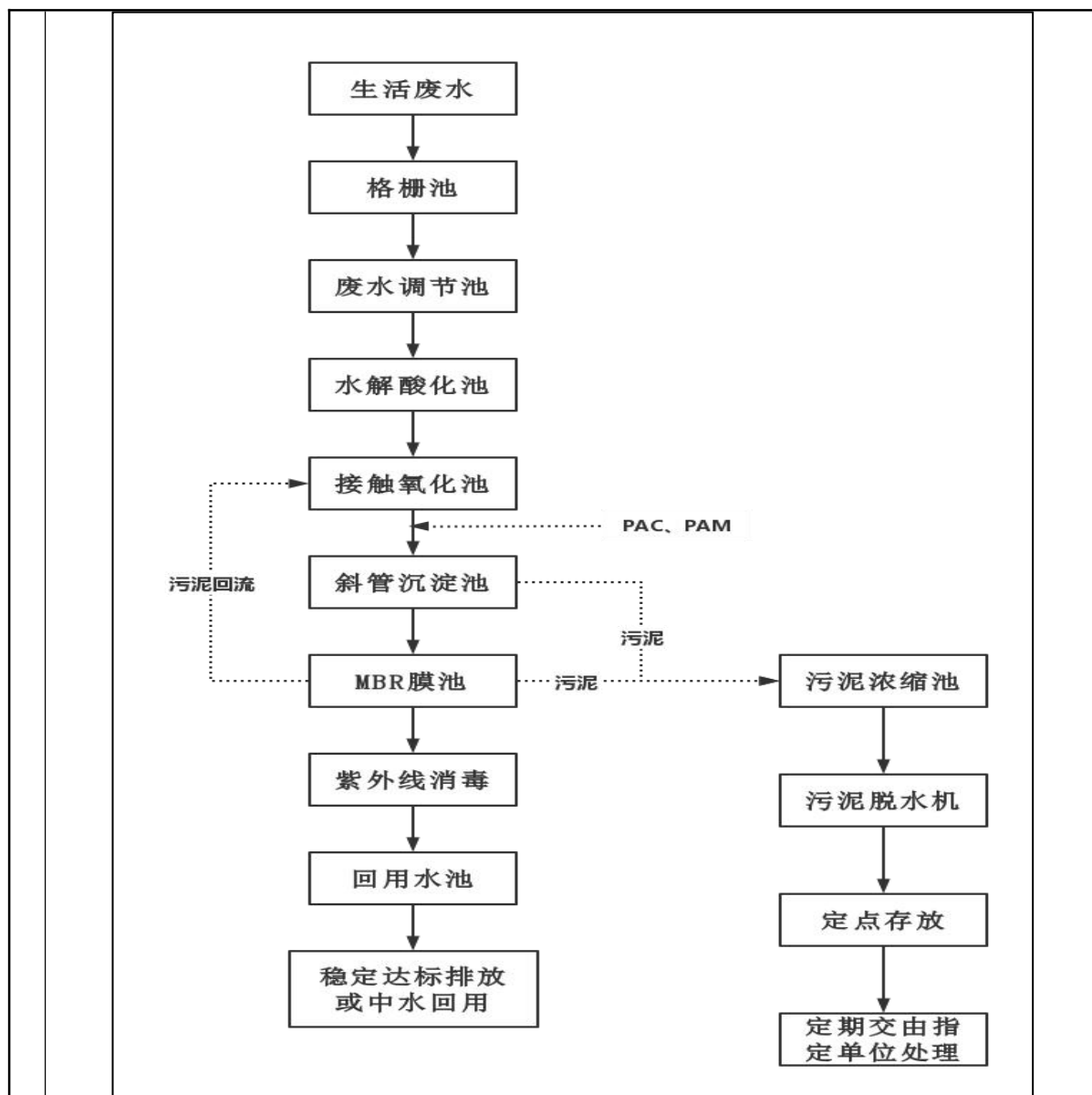
图 4-1 园区中水处理站生活污水处理工艺流程
