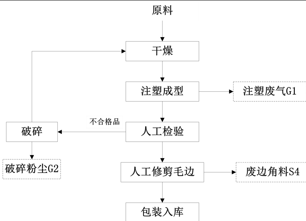
图 2-4 塑料配件工艺流程图
