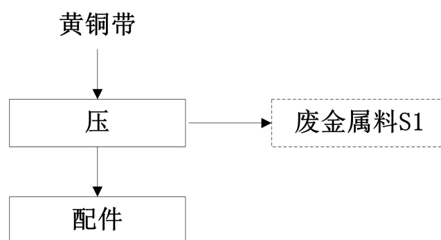
图 2-5 金工配件工艺流程图
