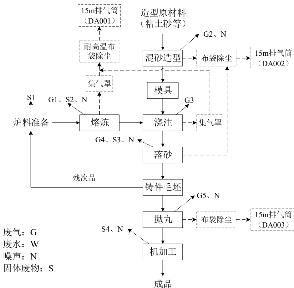
图 2-1 本次技改后生产工艺流程及产污节点图
