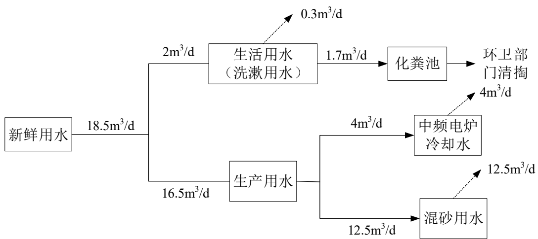
图 2-2 本次技改完成后全厂水平衡图
