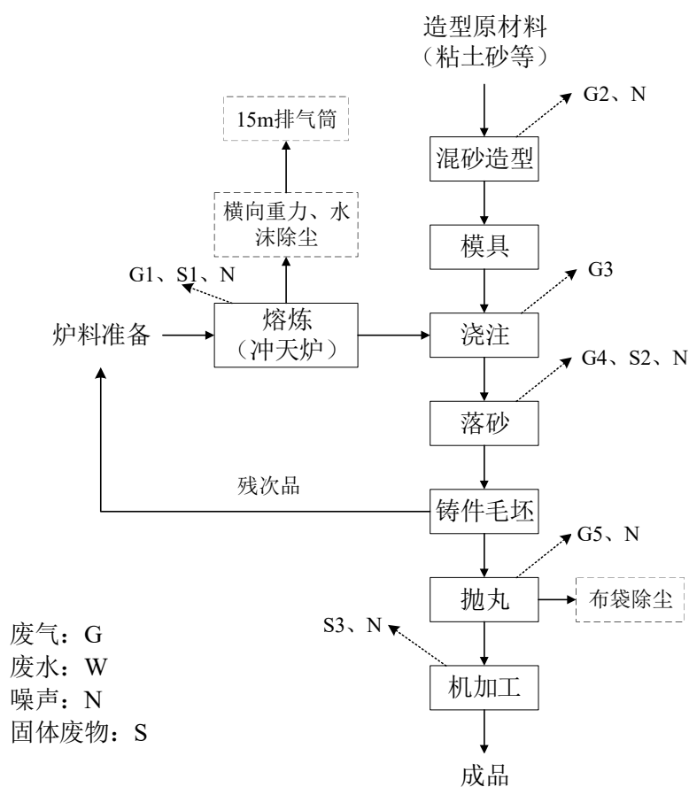
图 2-2 原有项目生产工艺及产污节点图
